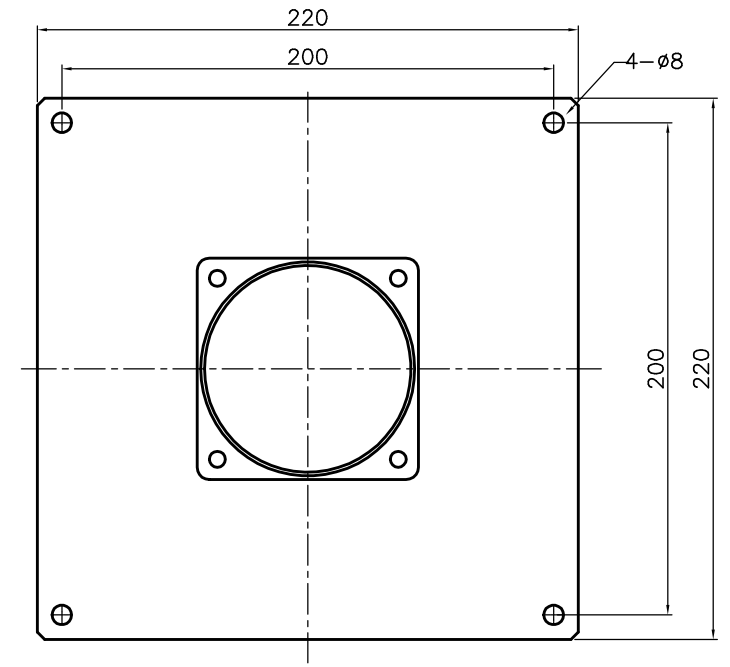
평면도(위에서 봄)
