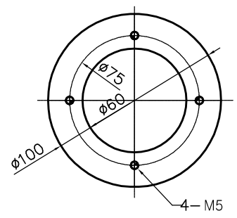
흡입구 상세도
